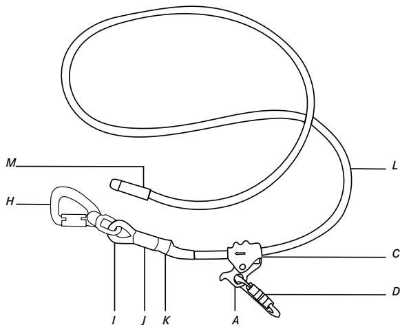
Extreme XP II (EN 358)
